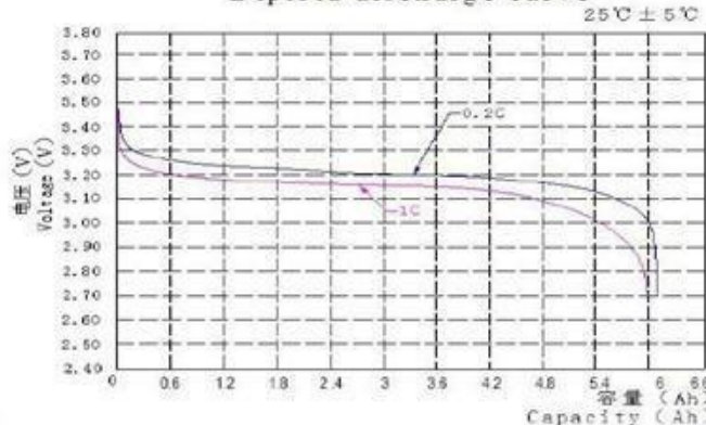
放电曲线图 Diploid discharge curve
