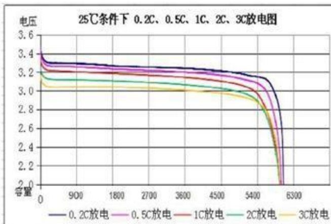
放电曲线图 Diploid discharge curve
