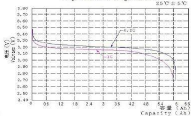
放电曲线图 Diploid discharge curve
